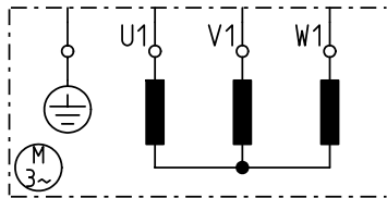
Sternschaltung/star wiring
