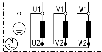
oder/ oder Dreieckschaltung/delta wiring
